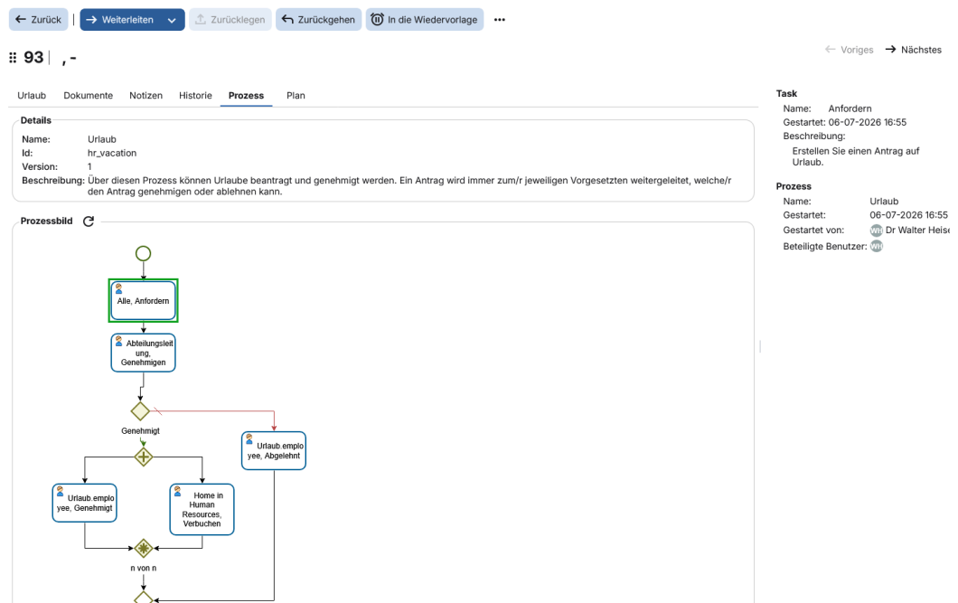
Abbildung 3.25: Prozessdefinition
