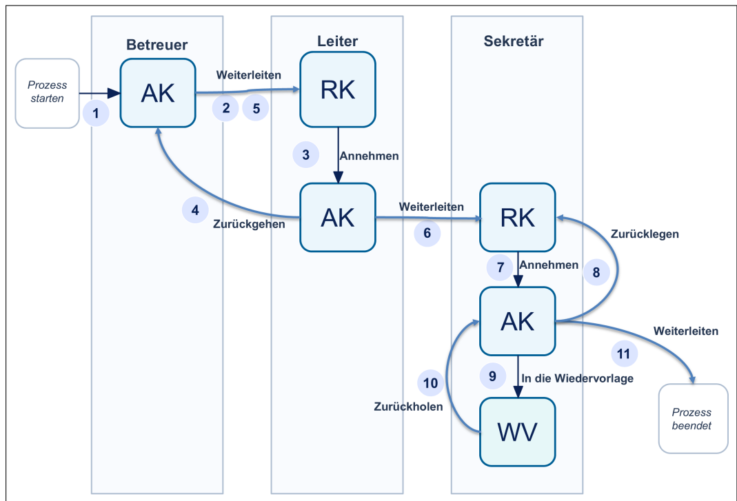
Abbildung 2.3: Workflow–Ablauf
